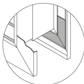
PARTICOLARE INSERIMENTO CONTROCORNICE
