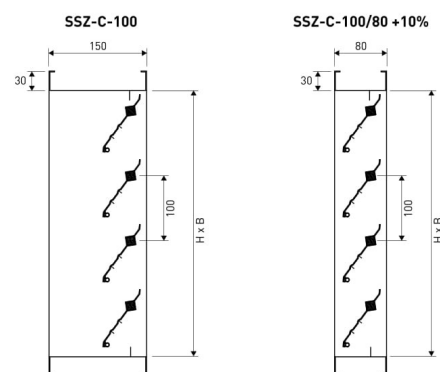
DISEGNI / DRAWINGS
