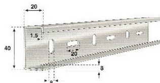
Profilo a C zincato forato 40x20x8 - sp. 20/10 barre da 4 m prezzo €
