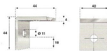
Angolare 90° per profilo a C 40x20 prezzo €
