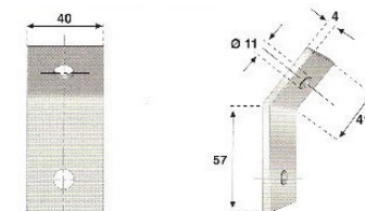
Angolare 45° per profilo a C 40x20 prezzo €
