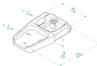
N 150 cerniera in nylon con foro ovale prezzo €/pz. N 152 cerniera in nylon con foro tondo prezzo €/pz.
