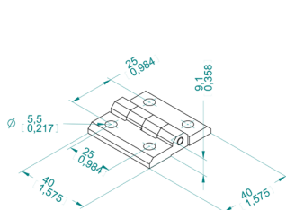
N 40x40 cerniera in nylon prezzo €/pz.
