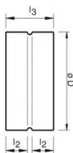
Manicotto femmina
